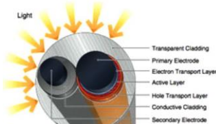
Napelemként működő szál (Konarka)
