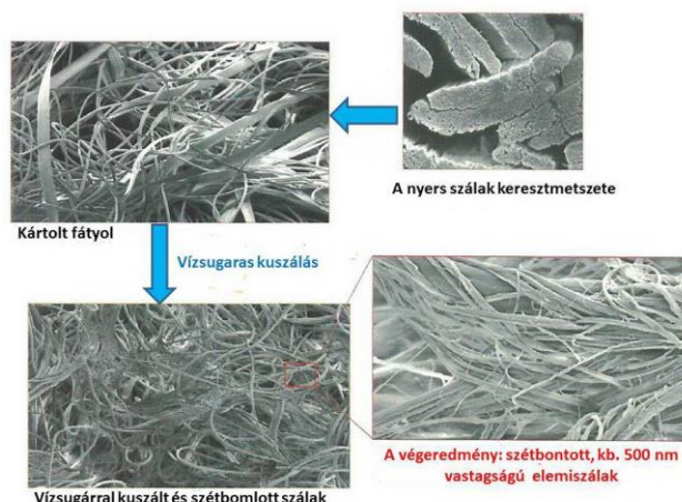
A Nanoacryl nemszött kelme kialakulása
